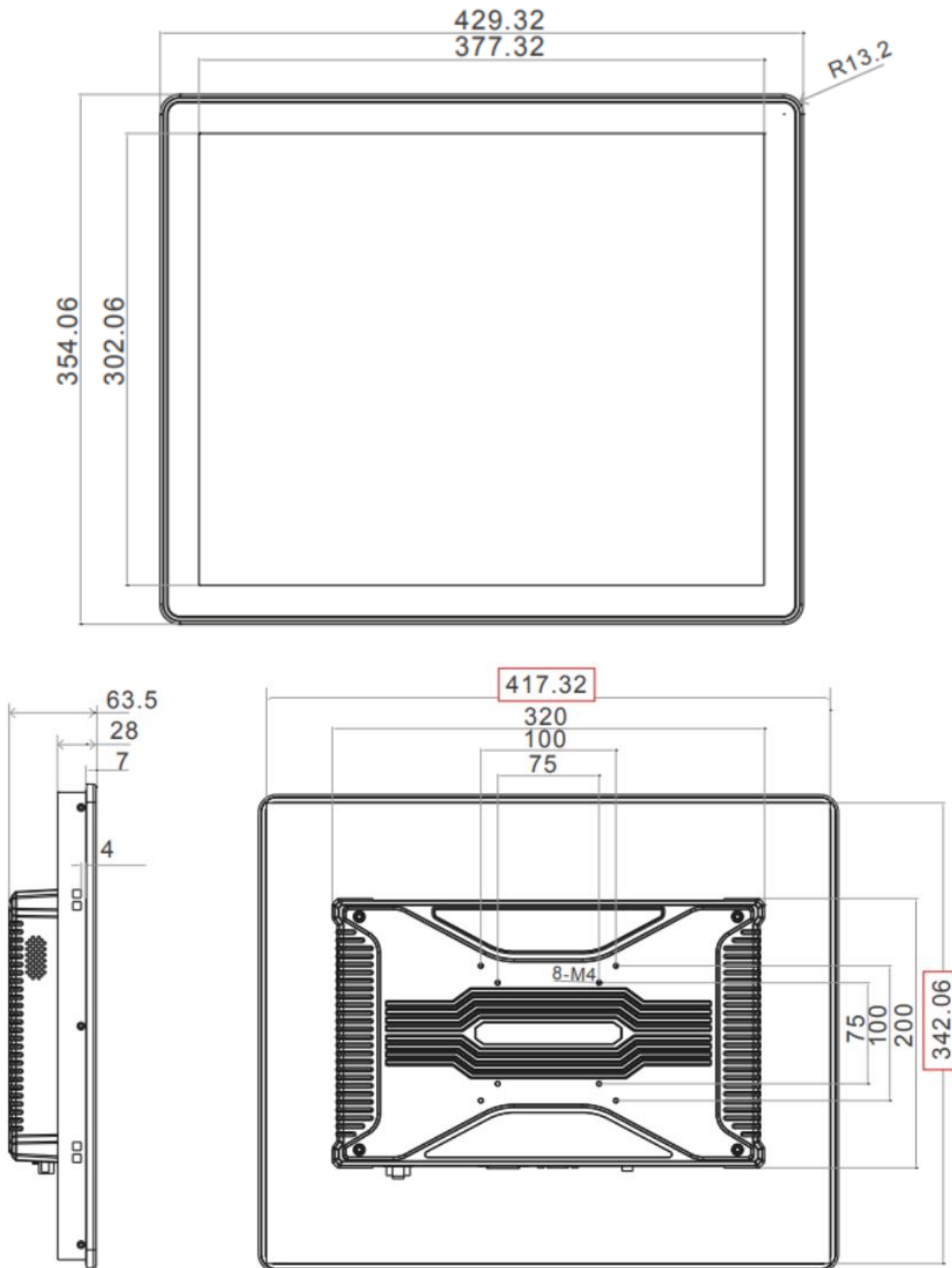
Размеры технологического выреза для панельного монтажа (ШхВ): 417,32x342,06 мм.
